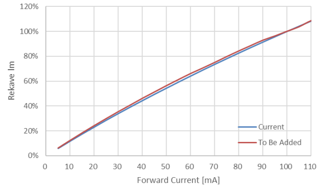
Lm (@25°C)
