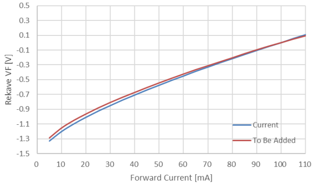
VF (@25°C)
