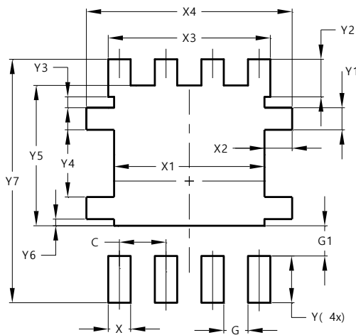
PowerDI5060-8
