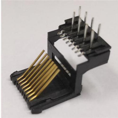
Material: PBT
